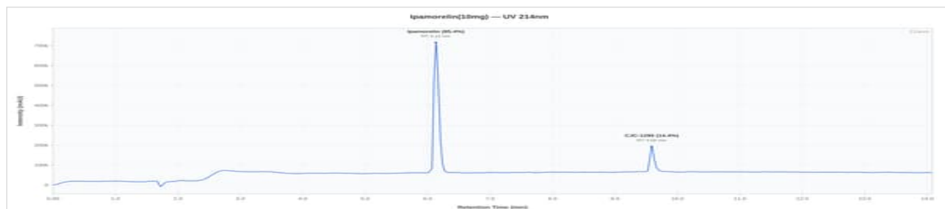
CJC-1295 / Ipamorelin 10mg - CJIP-A780: UV Chromatogram
